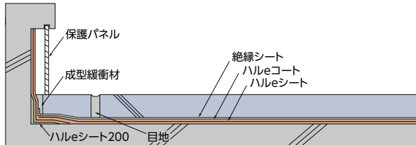
立上り露出/E-30C(A-1)
