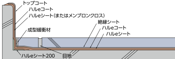
立上り露出/E-30C(A-1)
