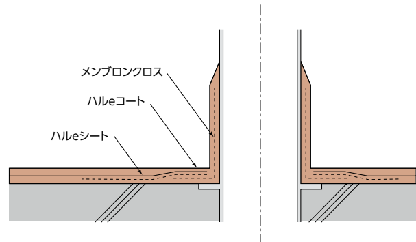
内部/E-30(E-1) 貫通パイプ廻り
